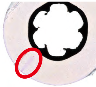
写真2 絶縁体の水トリ
