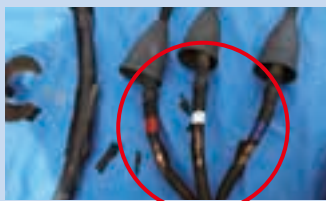
電柱側の高圧ケーブル端末処理部分
